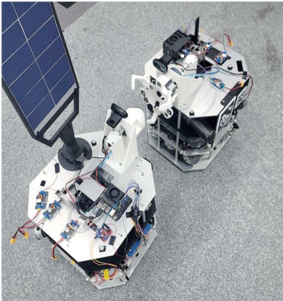
2대의 모사된 인공위성을 활용한 상대 항법 및 궤도 제어를 위한 지상 시뮬레이터
